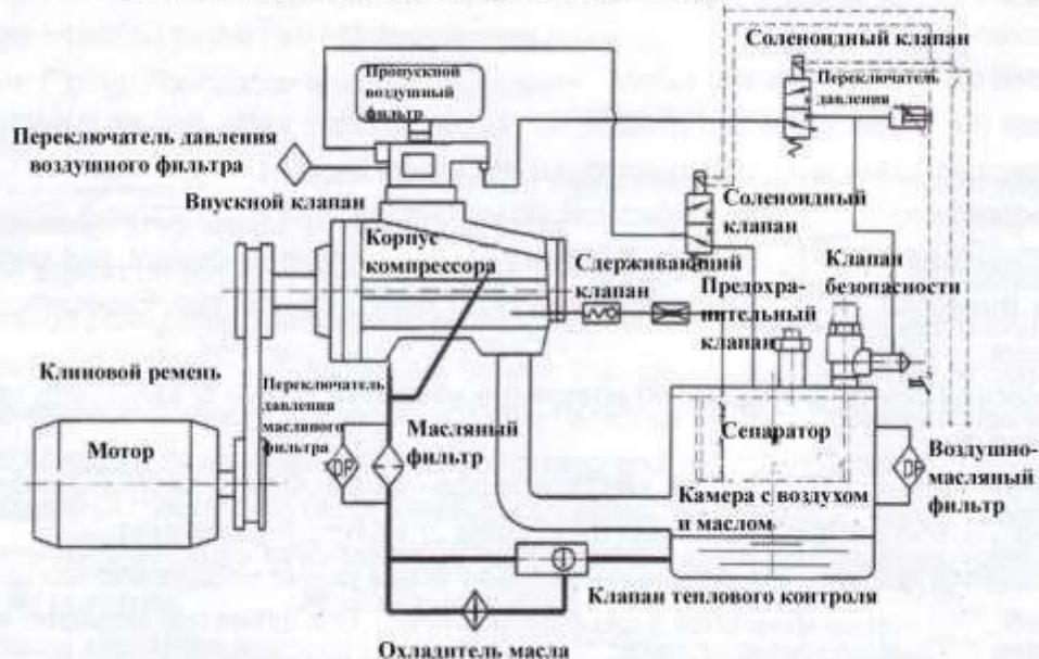
Схема технологического процесса (30 кВт)
